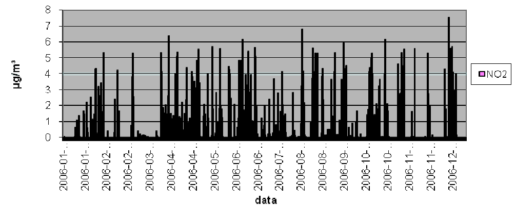
Azoto dioksido koncentracija, 1 val.
