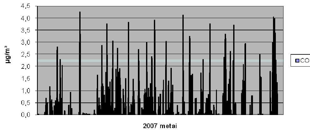
Anglies monoksido koncentracija, 8 val. vidurkis
