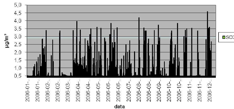
Sieros dioksido koncentracija, 1 val.
