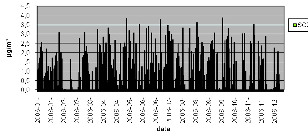
Sieros dioksido koncentracija, 1 val.
